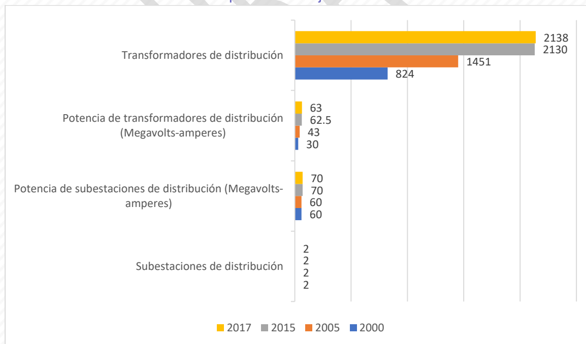
Gráfica 3. Unidades y potencia del equipo de transmisión y distribución de energía eléctrica del Municipio de Guanajuato de 2000 – 2017.
