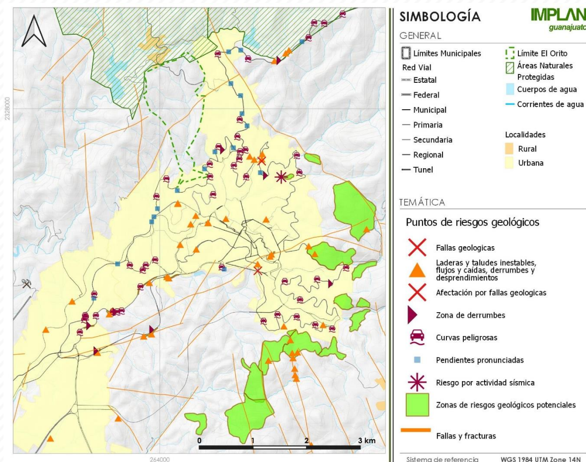
Mapa 23. Detalle zona de La Cañada Riesgos Geológicos.
